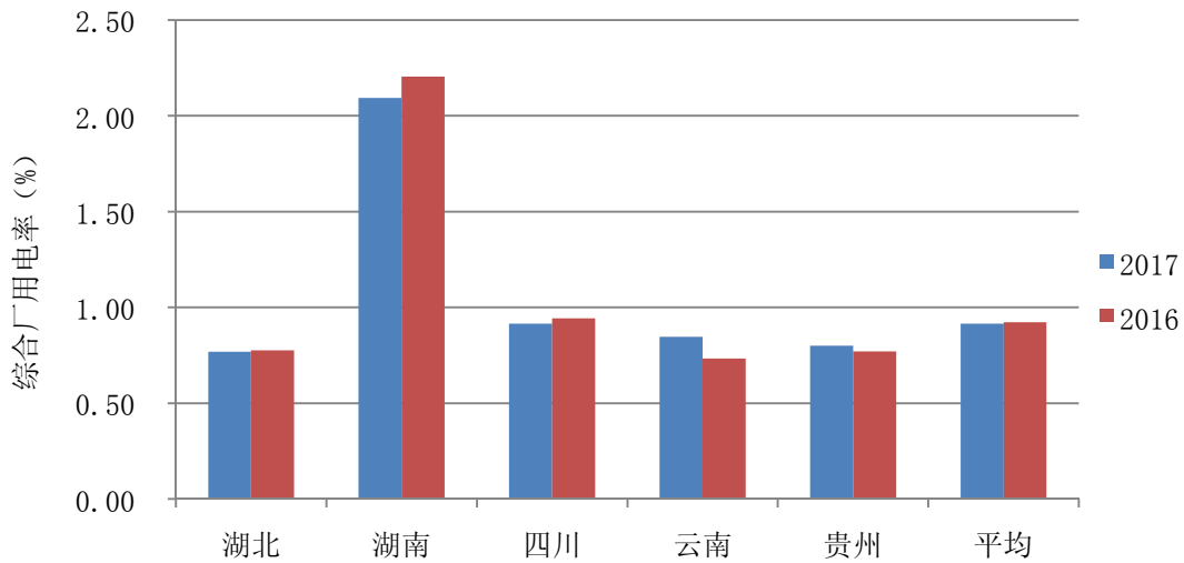
图 1-2 重点省份水电机组综合厂用电率
