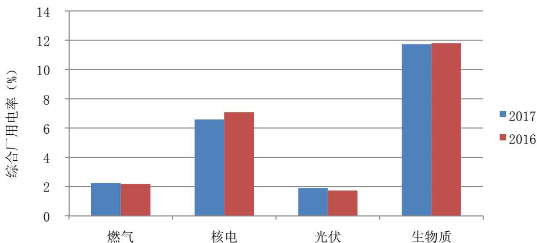
图 1-4 其他机组综合厂用电率
