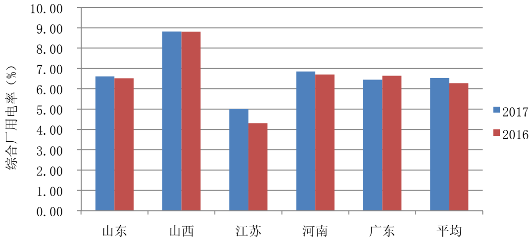
图 1-1 重点省份燃煤机组综合厂用电率
