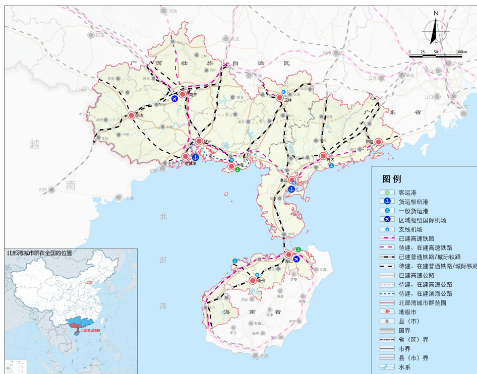
图 5 北部湾城市群综合交通规划图
